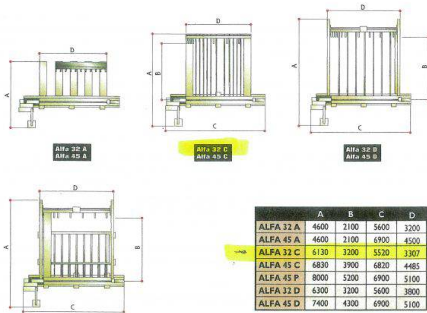
DIMENSIONI D'INGOMBRO / OVERALL DIMENSIONS
